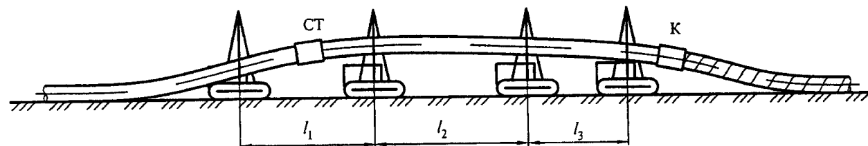
Рисунок 18. Схема расстановки трубоукладчиков для укладки плети газопровода при использовании комбайна для очистки и изоляции труб диаметром: а - 500 мм и менее; б - 700 - 1000 мм; в - 1000 - 1200 мм
