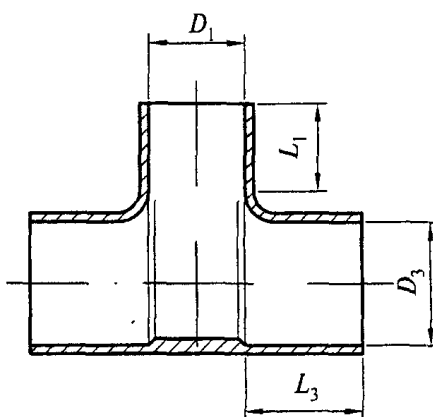
Рисунок Д.6. Тройник переходный
