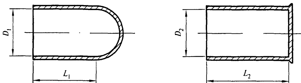
Рисунок Д.7. Заглушки
