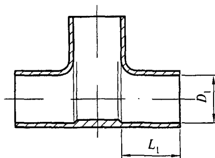
Рисунок Д.5. Тройник равнопроходный
