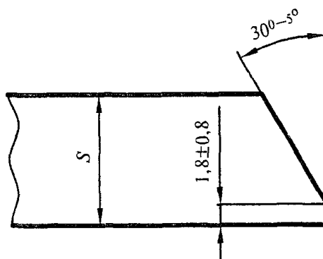
Рисунок 9. Схема обработки кромки
