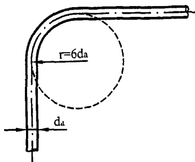
Рисунок 13. Холодная гибка медной трубы
